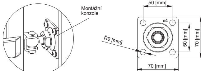
Obr. 6. Branka - standardní typ montáže B.
