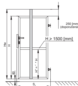
Obr. 15. Schéma konstrukce branky bez výplně - pohled z ulice.
