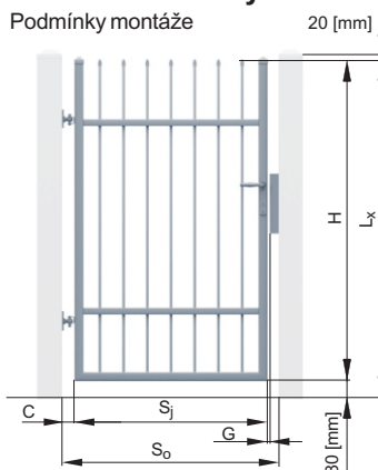
Obr. 7. Montážní rozměry potřebné pro správný výběr branky a její správnou montáž - pohled z pozemku.
